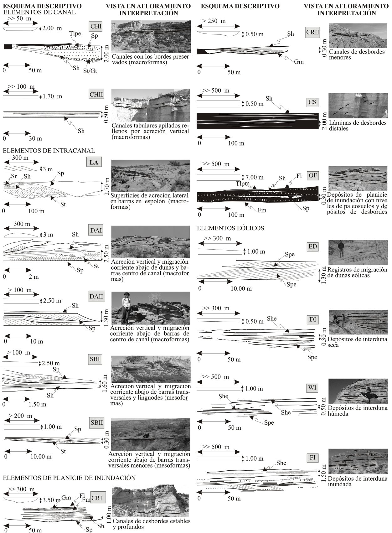
Figura 5. Cuadro de descripción de elementos arquitecturales ilustrado con esquemas y fotos de las mismas. Figure 5. Description of the architectural elements illustrated with schemes and pictures.
