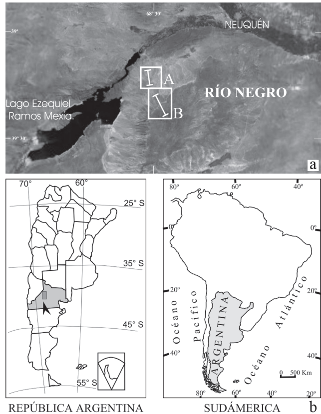
Figura 1. a y c) Mapa geológico e imagen satelitaria con la ubicación del área de trabajo. b y d) Imágenes Satelitarias con detalle del sector relevado.
