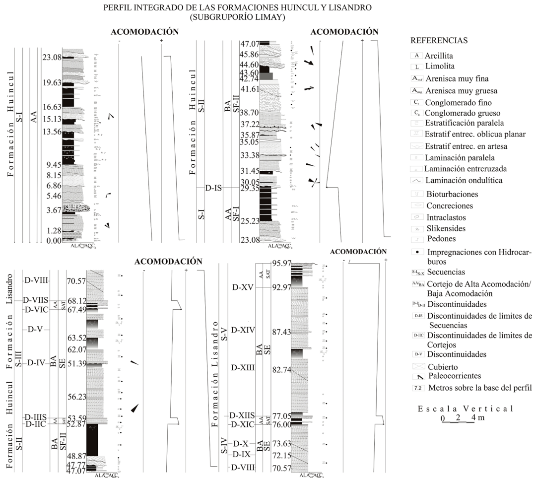
Figura 8. Perfil sintético con la definición de los cortejos para el Subgrupo Río Limay en el área de estudio. Figure 8. Schematic profile with the definition of the System Tracks (cortejos) for Río Limay Subgrupo for the study area.
