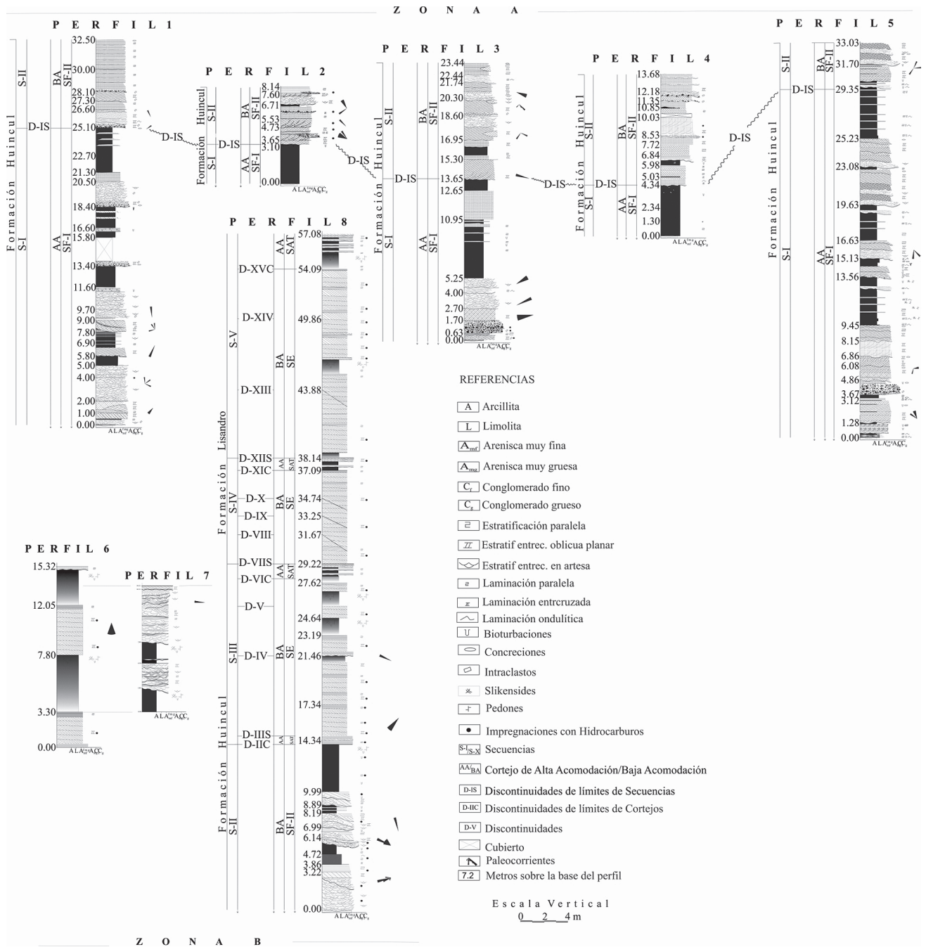
Figura 3. Perfiles estratigráficos del Subgrupo Río Limay en el departamento El Cuy (Río Negro). Figure 3. Stratigraphic profiles of the Río Limay Subgroup in the El Cuy Department (Río Negro).
