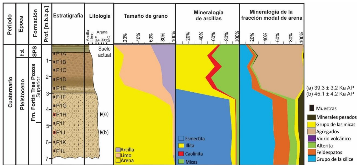
Figura 3. Sedimentología de la sección P1 R77.
