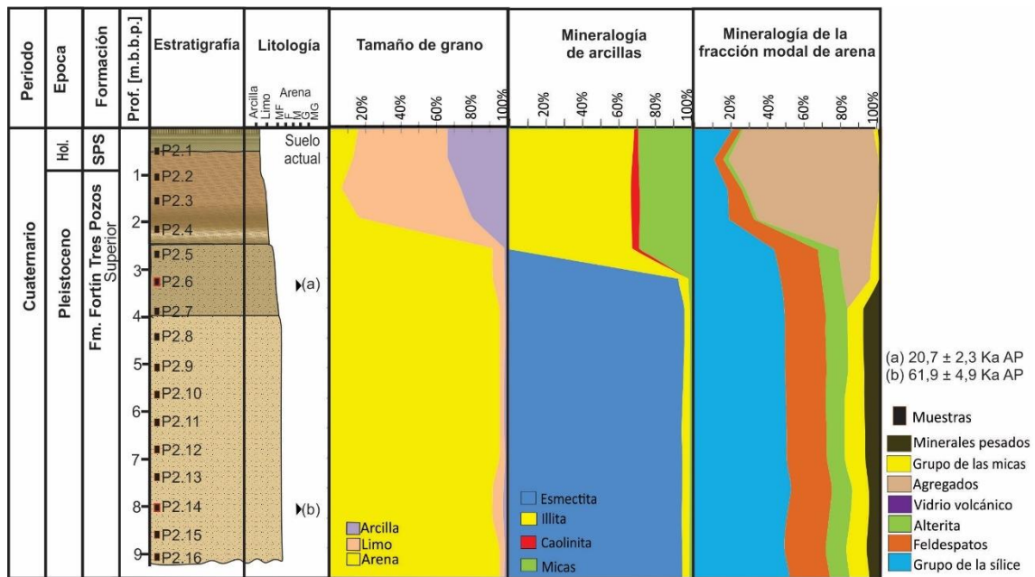
Figura 5. Sedimentología de la sección P2 VM.
