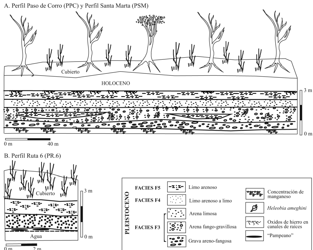
Figura 6. Perfiles en las barrancas entre Paso de Corro- Santa Marta (a) y Puente Ruta 6 (b). Figure 6. Cutbank profile between Paso de Corro - Santa Marta (a) and Puente Ruta 6 (b).
